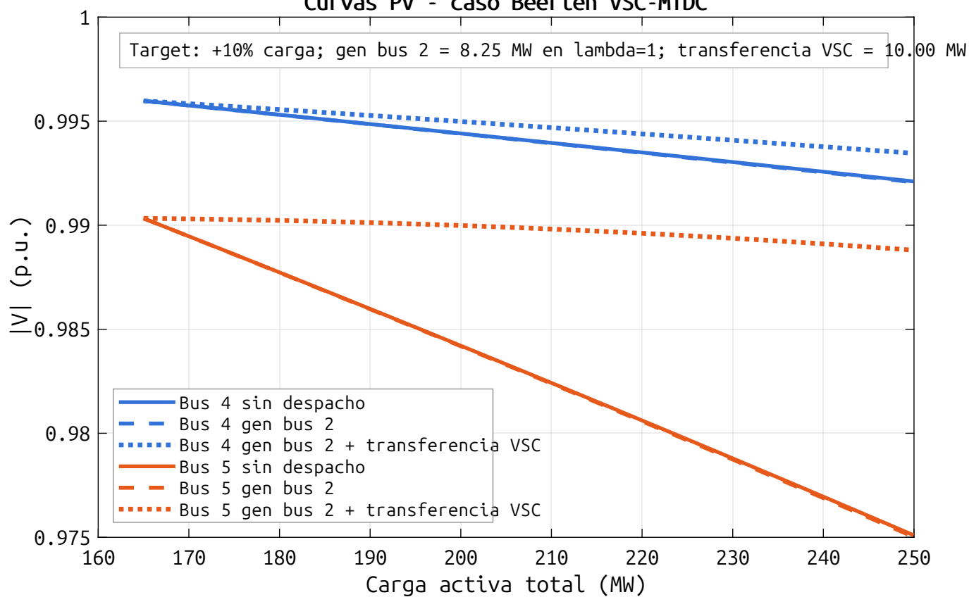
Curvas PV - caso Beerten VSC-MTDC
