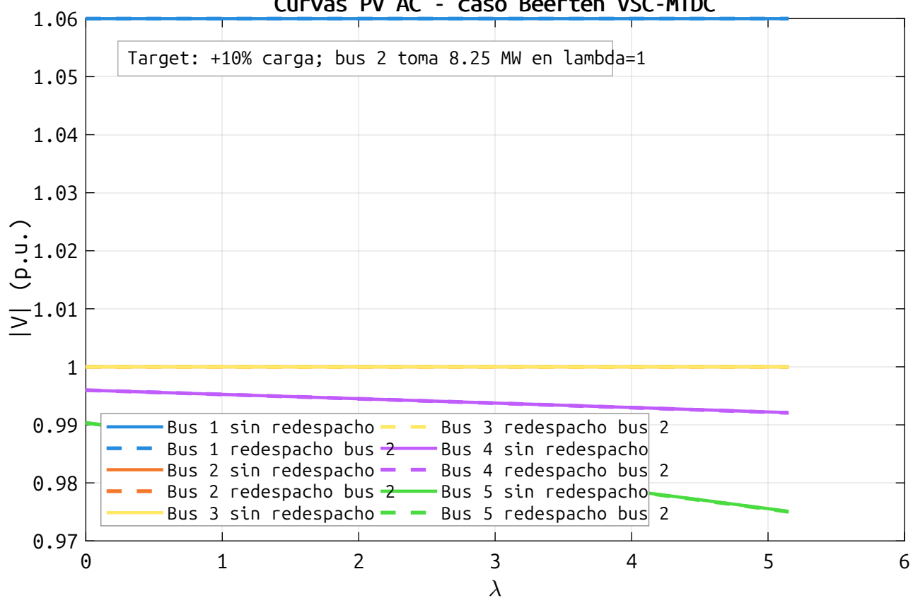
Curvas PV AC - caso Beerten VSC-MTDC
