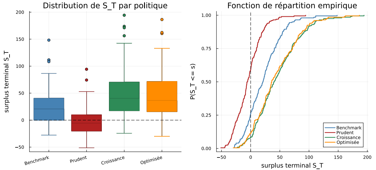
FIGURE 1 – Distribution du surplus terminal S_T par politique sur les 200 trajectoires hors échantillon : boîtes à moustaches colorées par politique (gauche) et fonctions de répartition empiriques (droite). Le trait pointillé marque le seuil S_T = 0 ; une ECDF évite l’étalement de masse de part et d’autre de zéro qu’induirait un noyau de densité.
