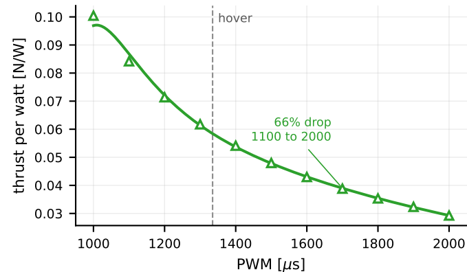
(d) propeller efficiency
