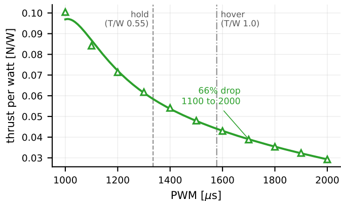
(d) propeller efficiency
