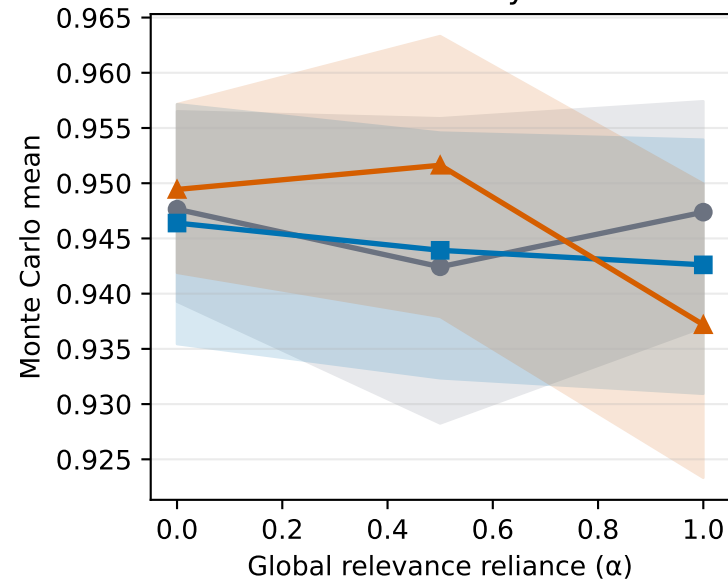
Plausibility
