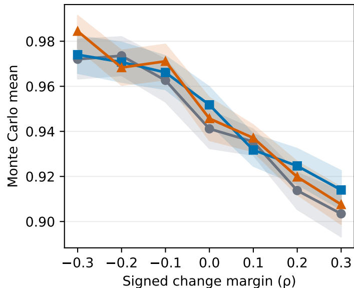
Plausibility
