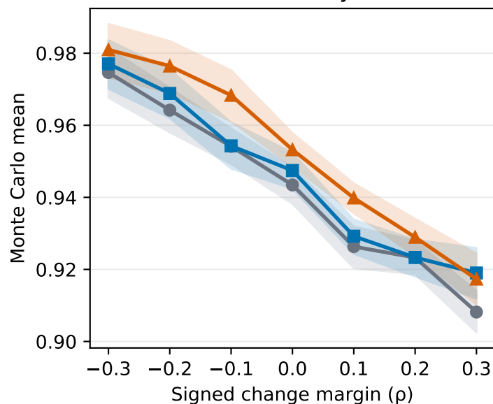
Plausibility
