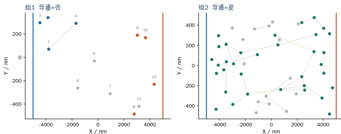
图 8 组 1、组 2 的接触图。节点取轴线中点，组 1 标注序号以便对照正文。青绿为跨越簇，蓝、橙为单侧簇，灰为孤立点，左右竖线为带电表面
