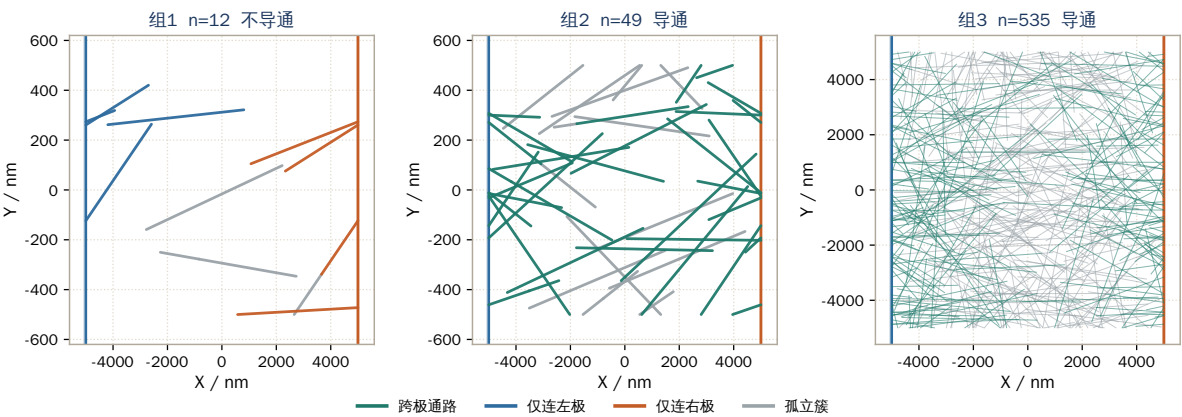
图 7 三组构型在 XY 平面上的通路着色。青绿为同时连通两极的跨越簇，蓝、橙为只接到单侧电极的簇，灰为孤立簇。左右竖线为带电表面
