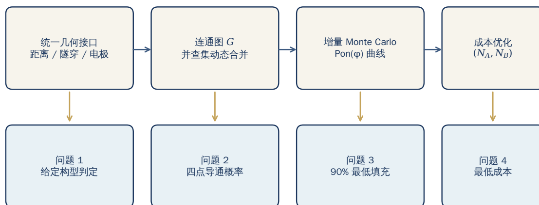
图 1 距离核与并查集在四问中的复用关系
