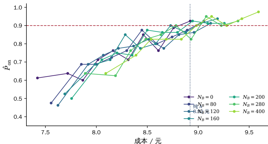
图 18 固定 N_B 时成本与导通概率的关系。水平虚线为 90% 约束, 竖虚线为纯 A 成本
