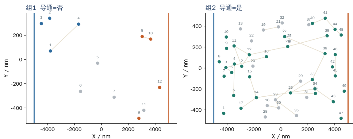
图 8 组 1、组 2 的接触图（节点取轴线中点）。青绿为跨越簇，蓝、橙为单侧簇，灰为孤立点；左右竖线为带电表面
