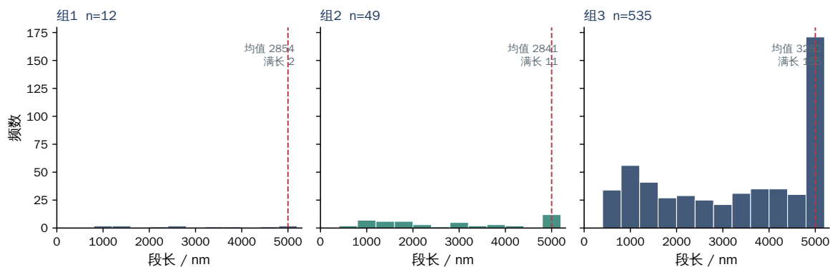
图 5 附件三组圆柱段的长度分布。虚线为母圆柱名义长度 5000 nm，其左侧的短段即边界截断的产物
