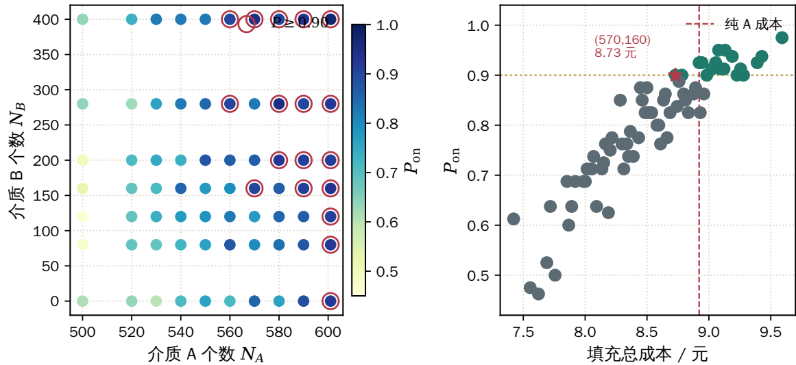
图 16 左: (N_A, N_B) 上的导通概率, 红圈为 \hat{P} \geq 0.90 的格点; 右: 成本-概率散点, 星号为网格内最低成本可行点
