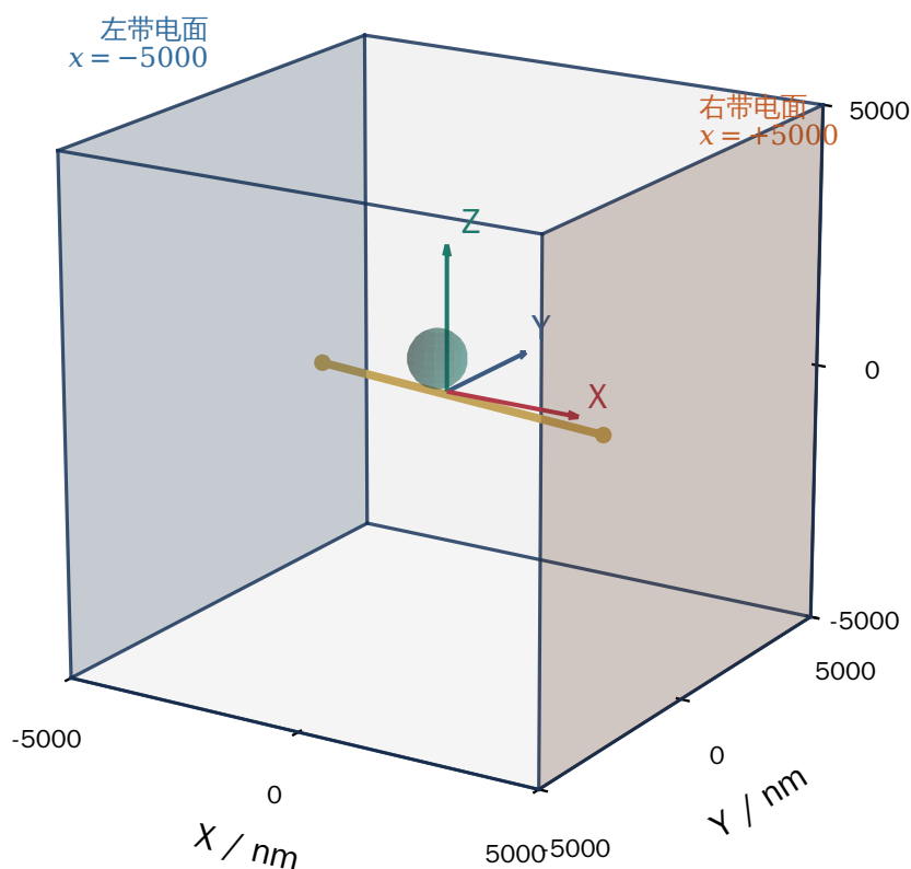
图2 微构体坐标系、左右带电面以及两类介质的相对尺度示意
