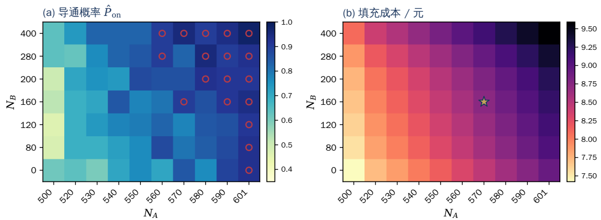
图 17 混合填充网格的矩阵视图。(a) 导通概率，红圈为 \hat{P} \geq 0.90 ；(b) 成本，金星为最低成本可行点
