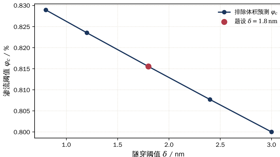
图 20 排除体积阈值随隧穿距离的变化。题设 \delta = 1.8 \text{ nm} 处曲线极为平缓
