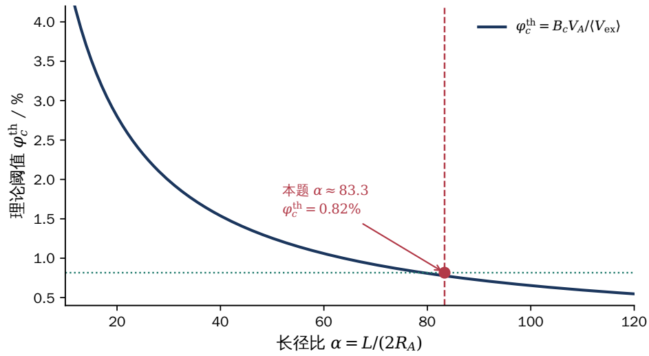
图 14 排除体积阈值随长径比的变化。红点为本题参数 \alpha \approx 83.3 , \varphi_c^{th} = 0.82\%
