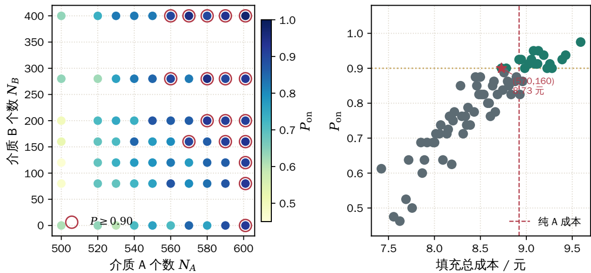
图 16 左: (N_A, N_B) 上的导通概率, 红圈为 \hat{P} \geq 0.90 的格点; 右: 成本-概率散点, 星号为网格内最低成本可行点
