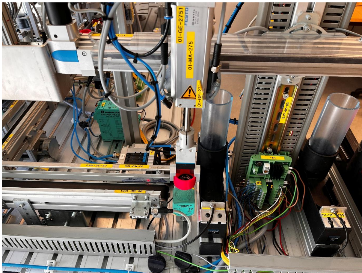
Figur 13 Kopper ved RFID-leser på handling-stasjonen.
