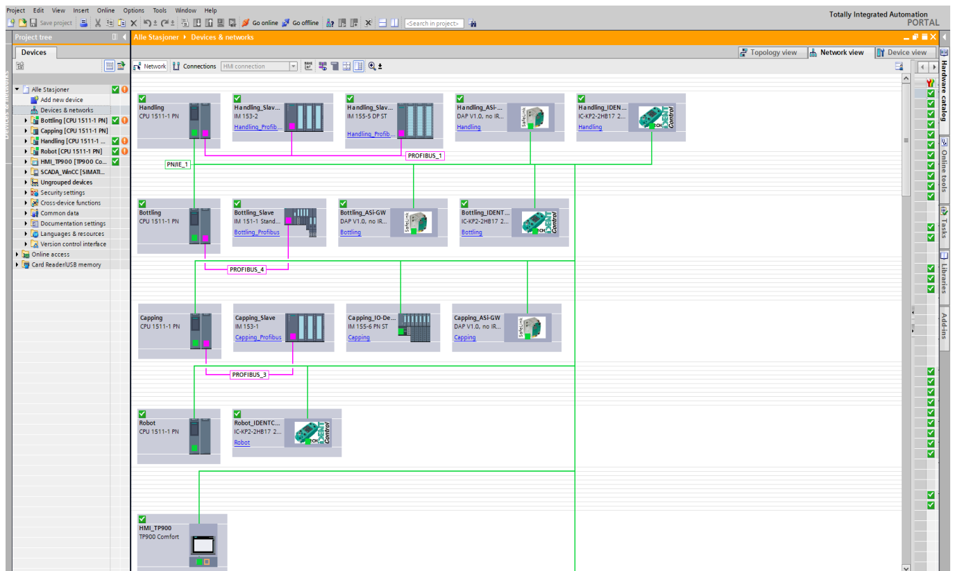
Figur 5 Skjerm bilde fra TIA Portal V17 med oversikt over alle komponenter.
