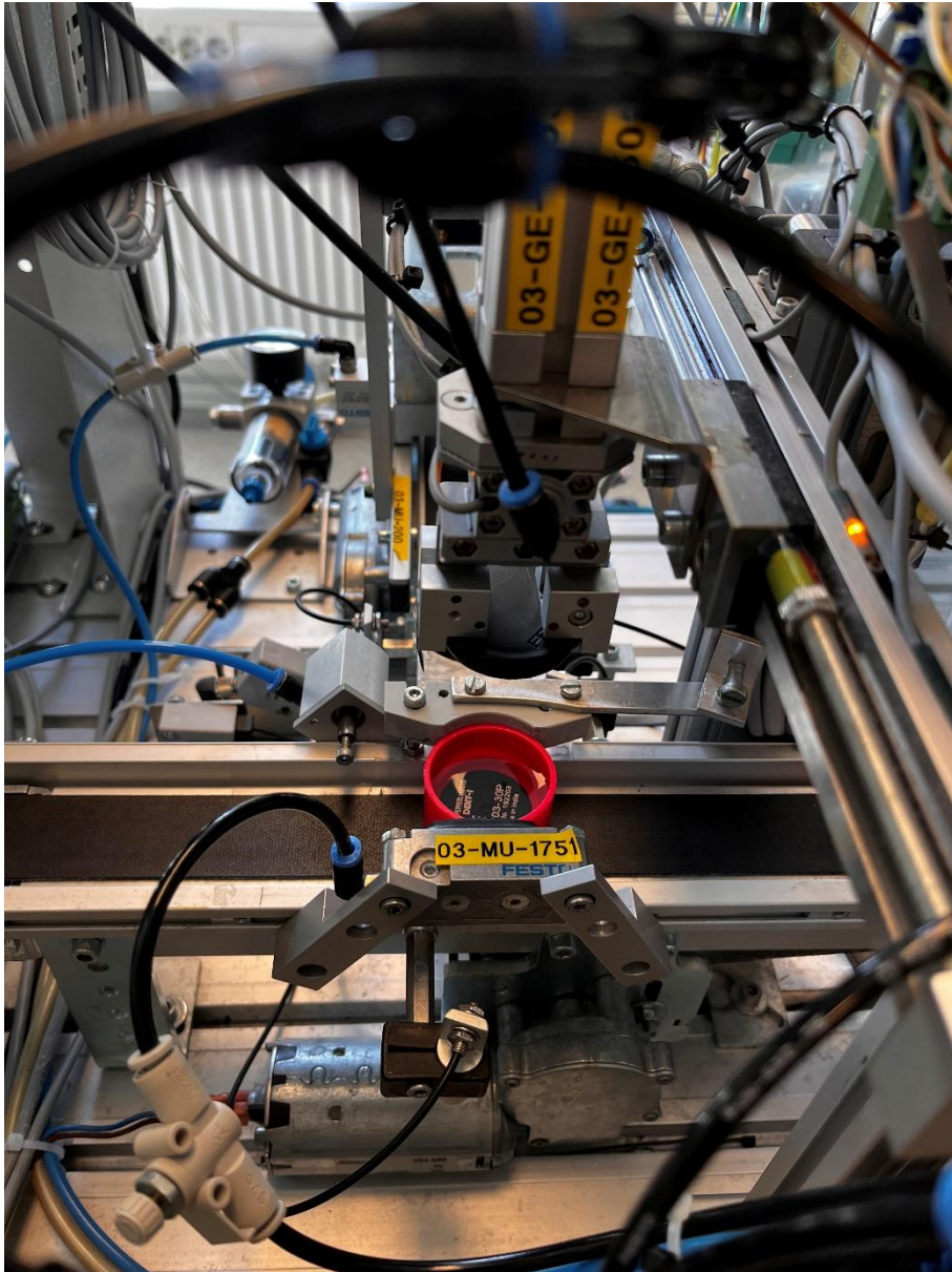
Figur 14 Kopp etter lukking.
