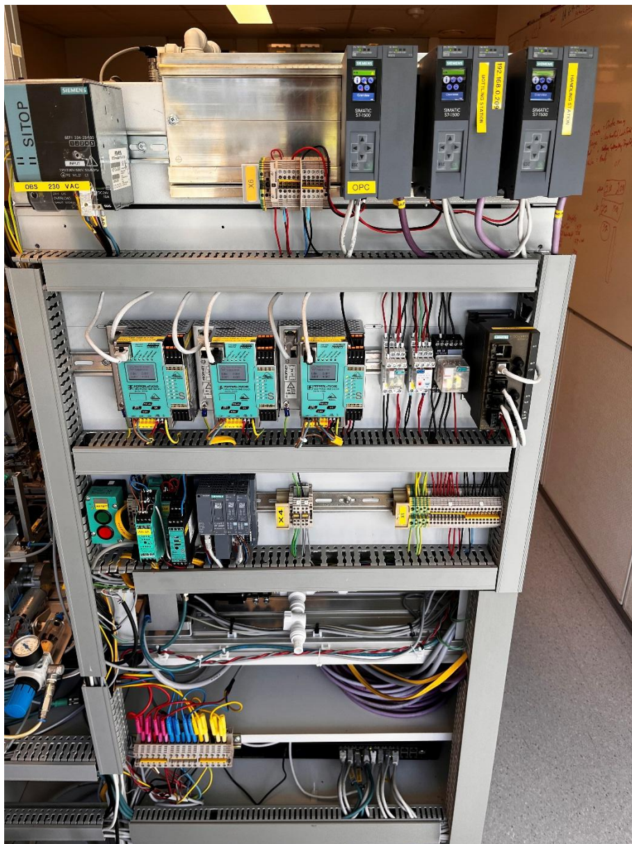
Figur 15 Bilde av PLS S7-1500, ASI Gateway, Safe link og Nettverk Switch helt ned
