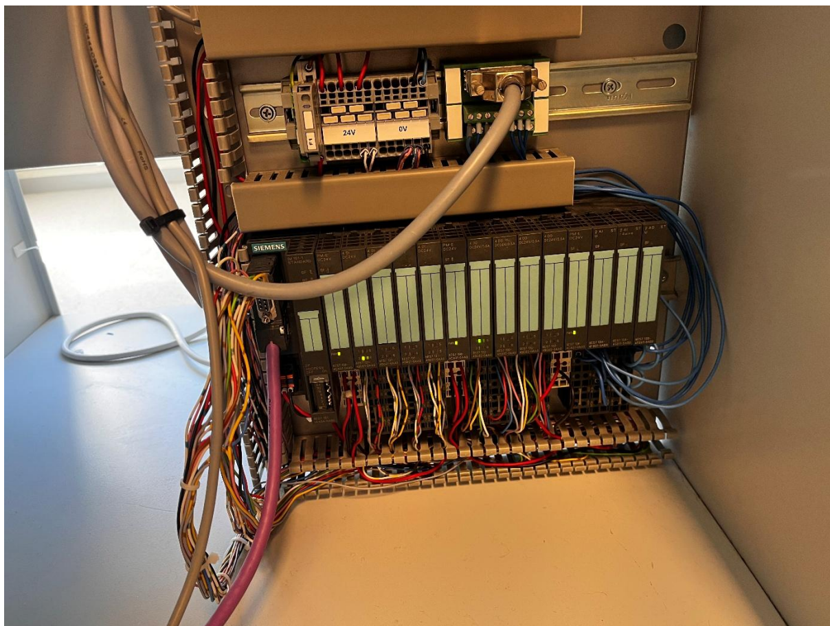
Figur 27 I/O-moduler til fylling-PLS.
