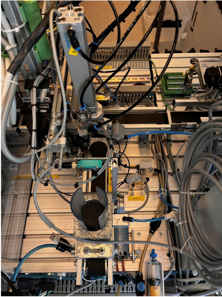
Figur 29 Capping-stasjon.
