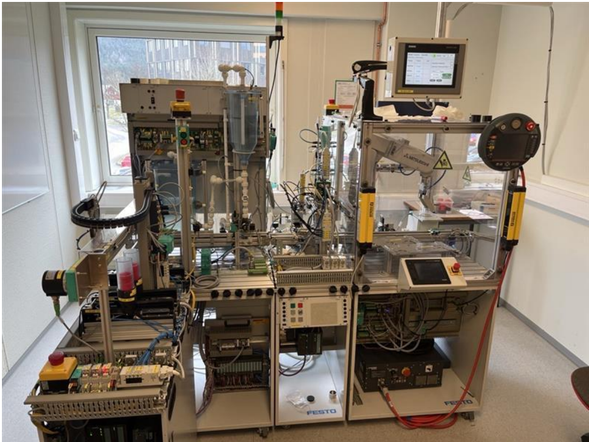
Figur 1 Festo anlegge
