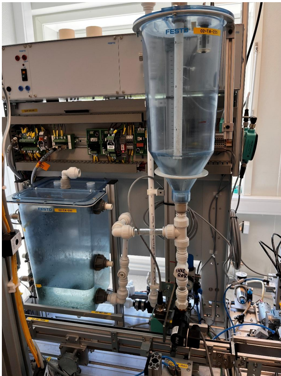
Figur 19 Tank til fylling.
