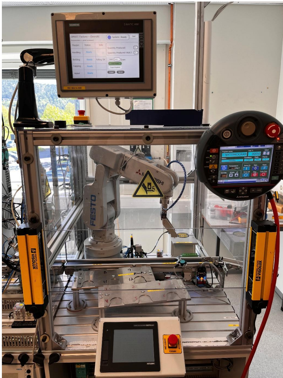
Figur 10 Robot Stasjon.
