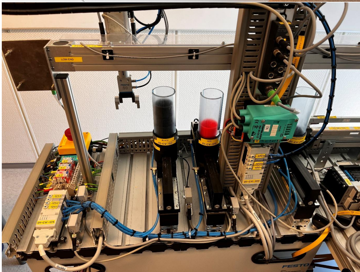
Figur 25 Handling-stasjon
