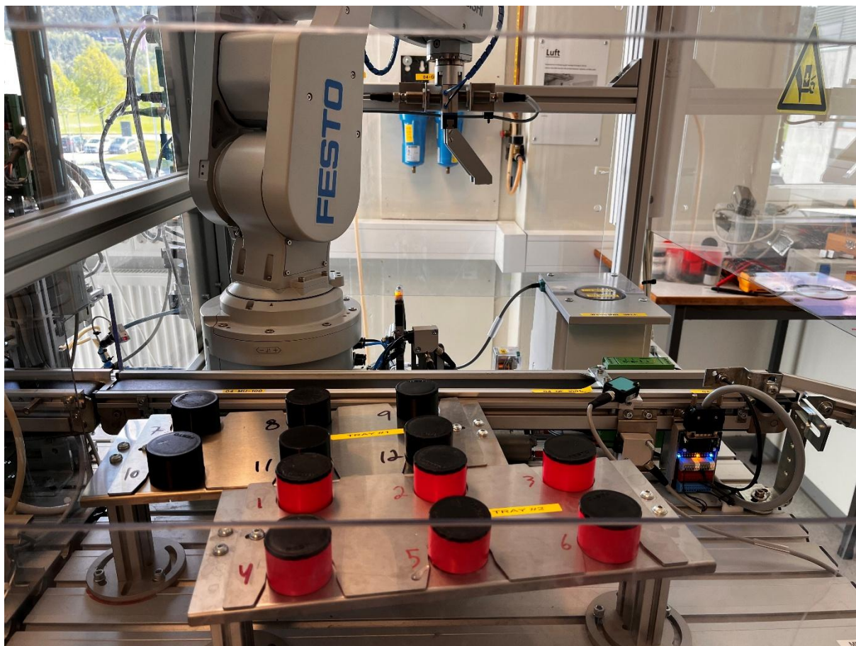
Figur 18 : Ferdig ordre med roboten i sikker posisjon.
