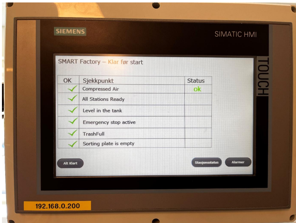
Figur 7 HMI som viser at anlegget er klart for start.
