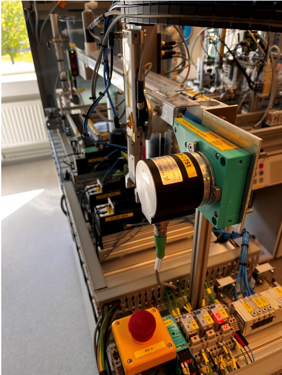
Figur 6 Bilde av enkoder på handling-stasjonen.
