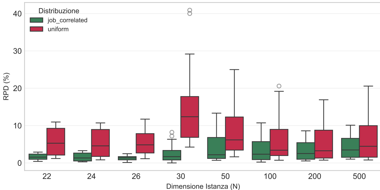
Relative Percentage Deviation (RPD) per Distribuzione (Istanze Grandi - Scalabilità Algoritmo)
