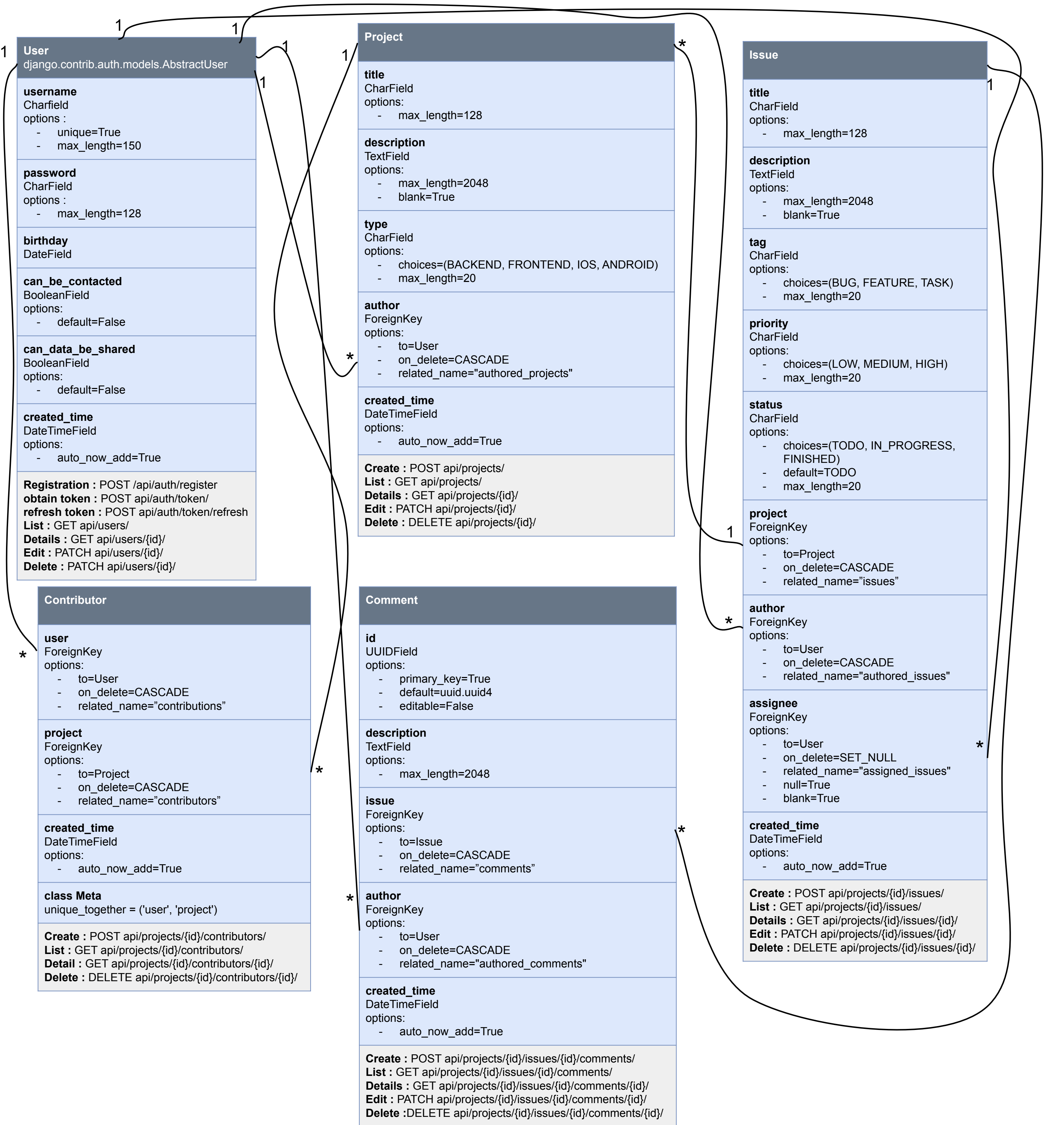
Diagramme Modèles SoftDesk
