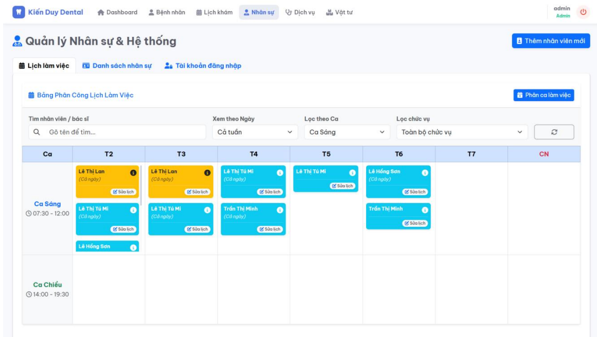
Hình 6.47 Giao diện Phòng khám - Tìm kiếm Lịch làm việc Nhân viên
