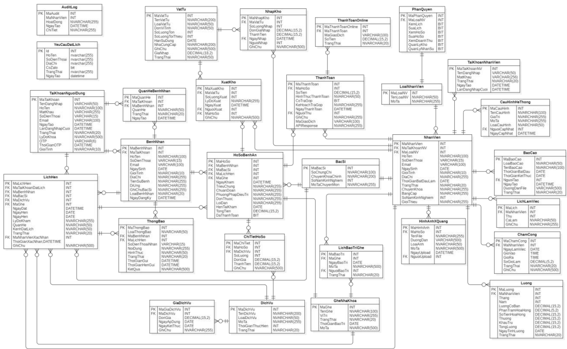
Hình 3.2 Sơ đồ ERD
