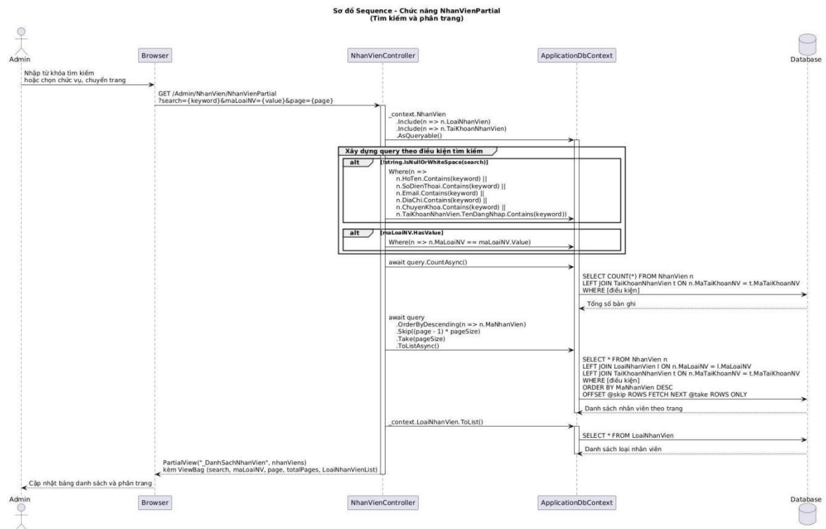
Hình 3.4 Sơ đồ Sequence Diagram – chức năng quản lý Nhân viên
