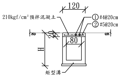
水泥板橋標準斷面圖 Scale=1:100
