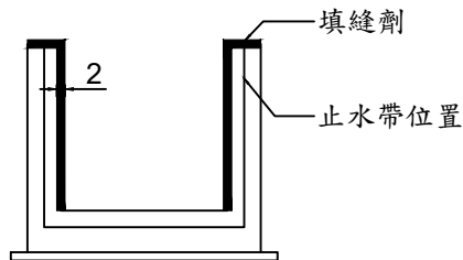
PVC止水帶斷面圖 Scale=N. T. S.
