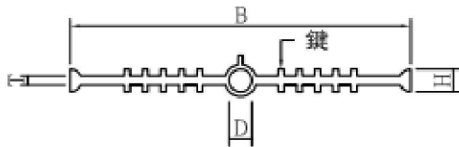
PVC止水帶示意圖 Scale=N. T. S.
