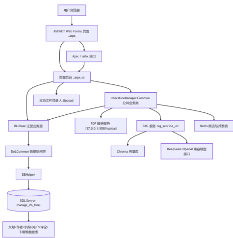
图 3-2 系统总体架构图
