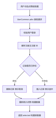
图 7-6 点赞收藏切换流程
