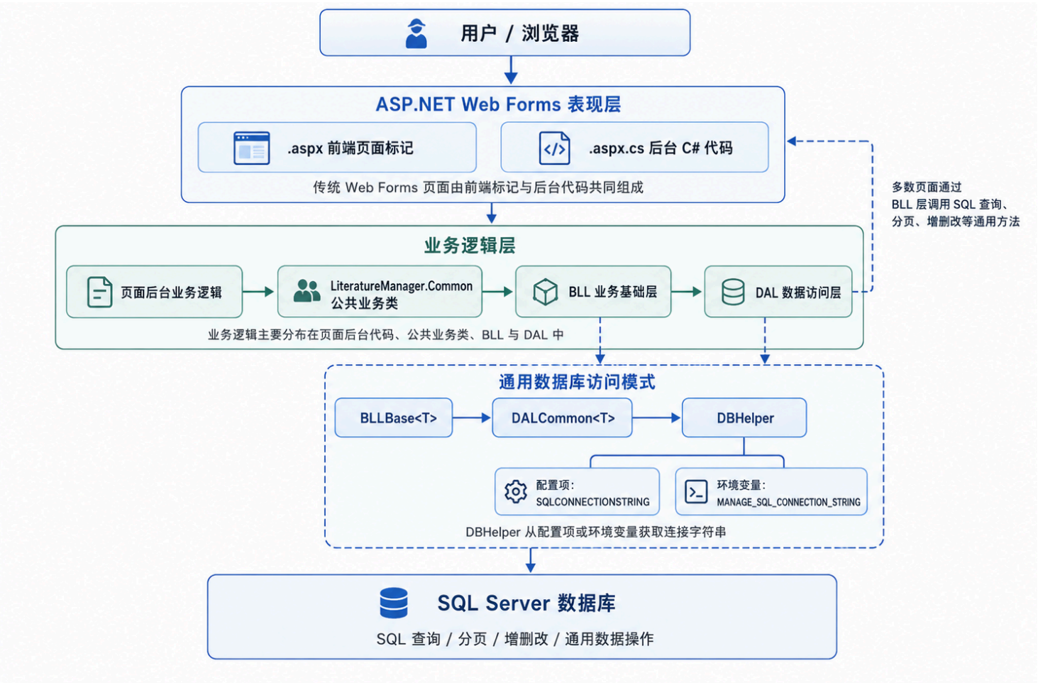
图 3-1 数据访问模式示意图
