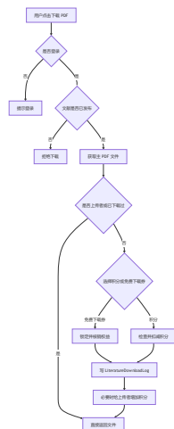
图 7-7 文件上传下载流程
