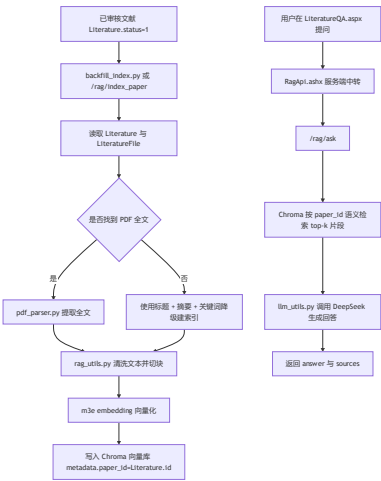
图 5-2 RAG 智能问答数据流
