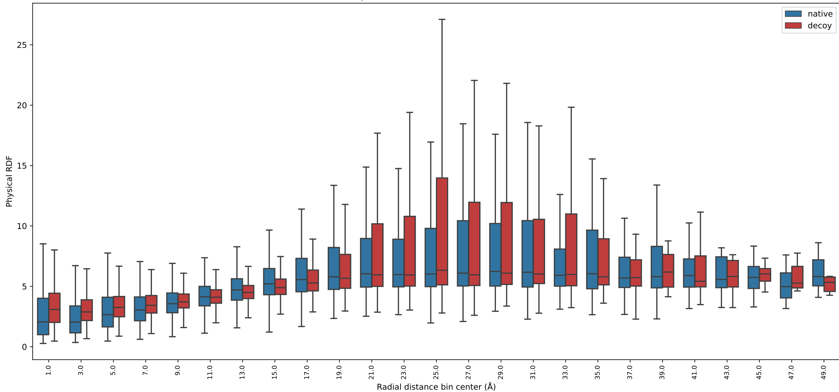
Physical RDF - actual radial distance
