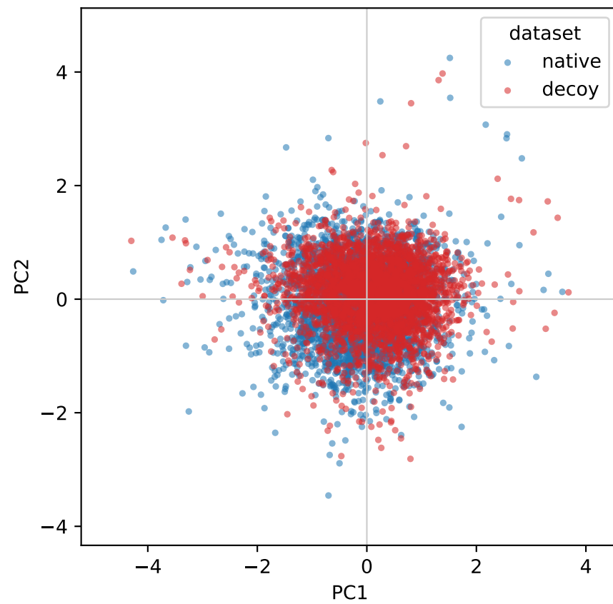
Zernike RDF
