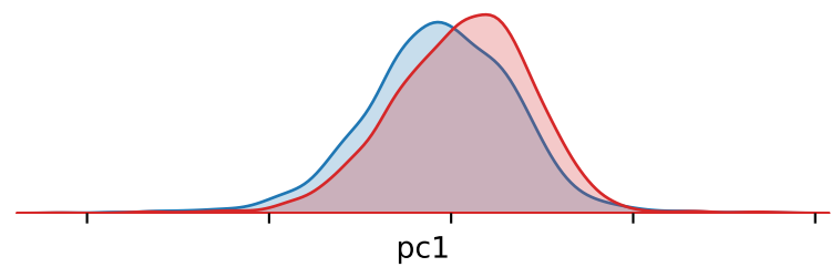
Zernike RDF
