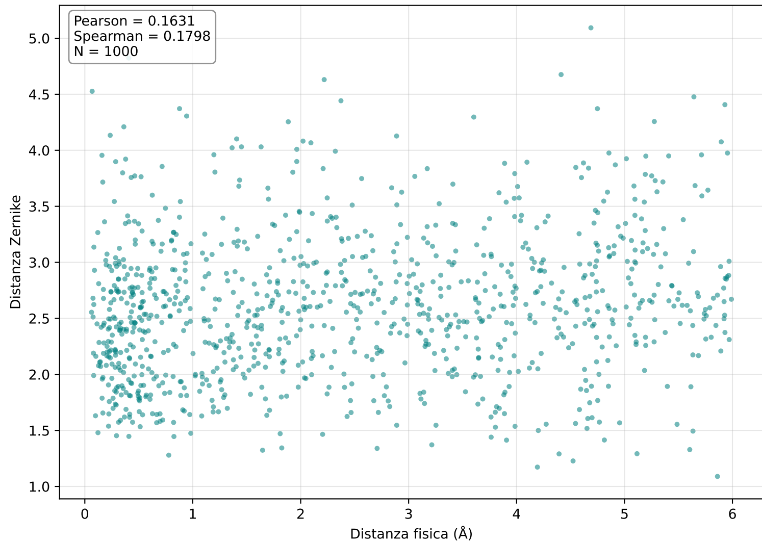
1A1U: distanza fisica vs distanza Zernike
