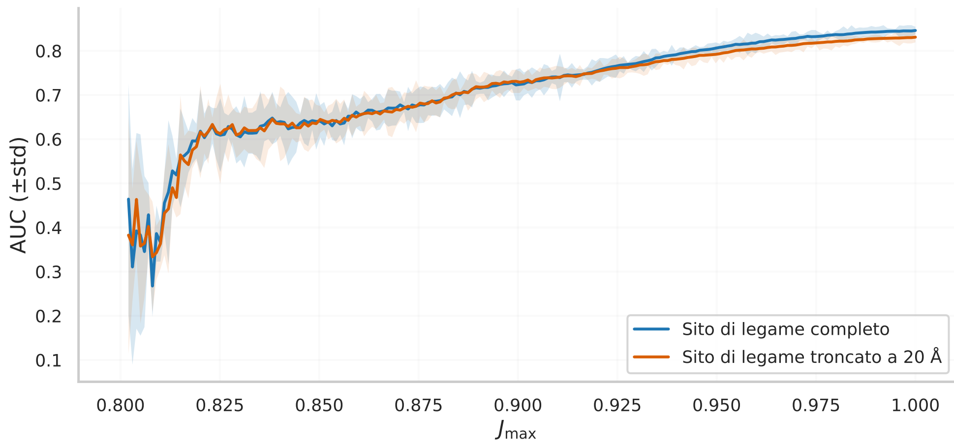
AUC vs J_{\max}
