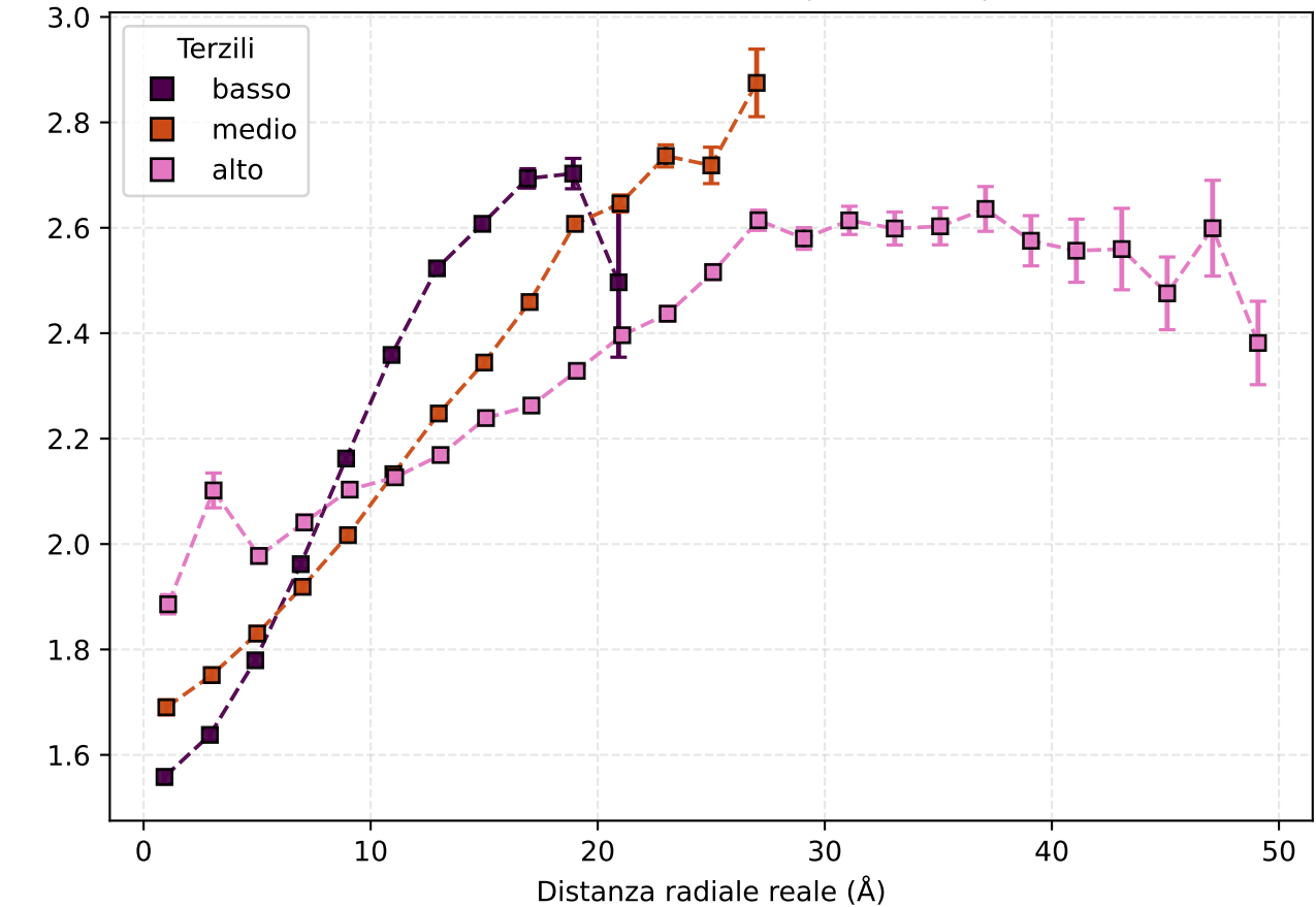
Distanza radiale reale (bin da 2 Å)
