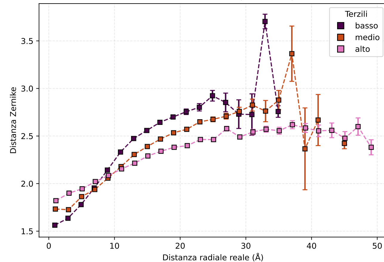
Distanza radiale reale (bin da 2 Å)
