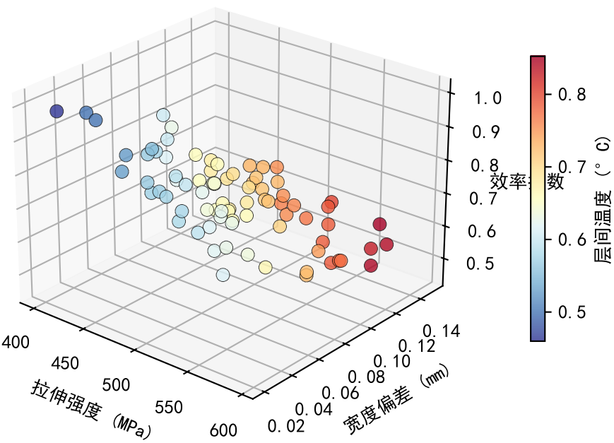
(c) 带优化偏好的帕累托前沿
