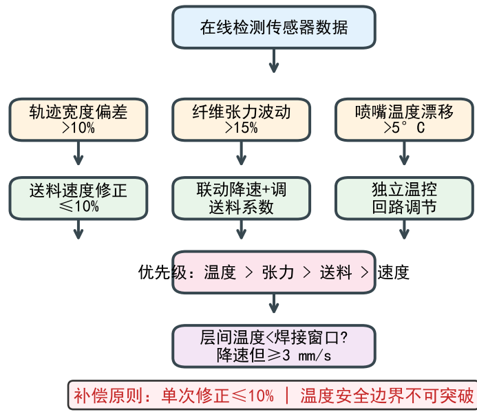
(d) 在线自适应补偿机制
