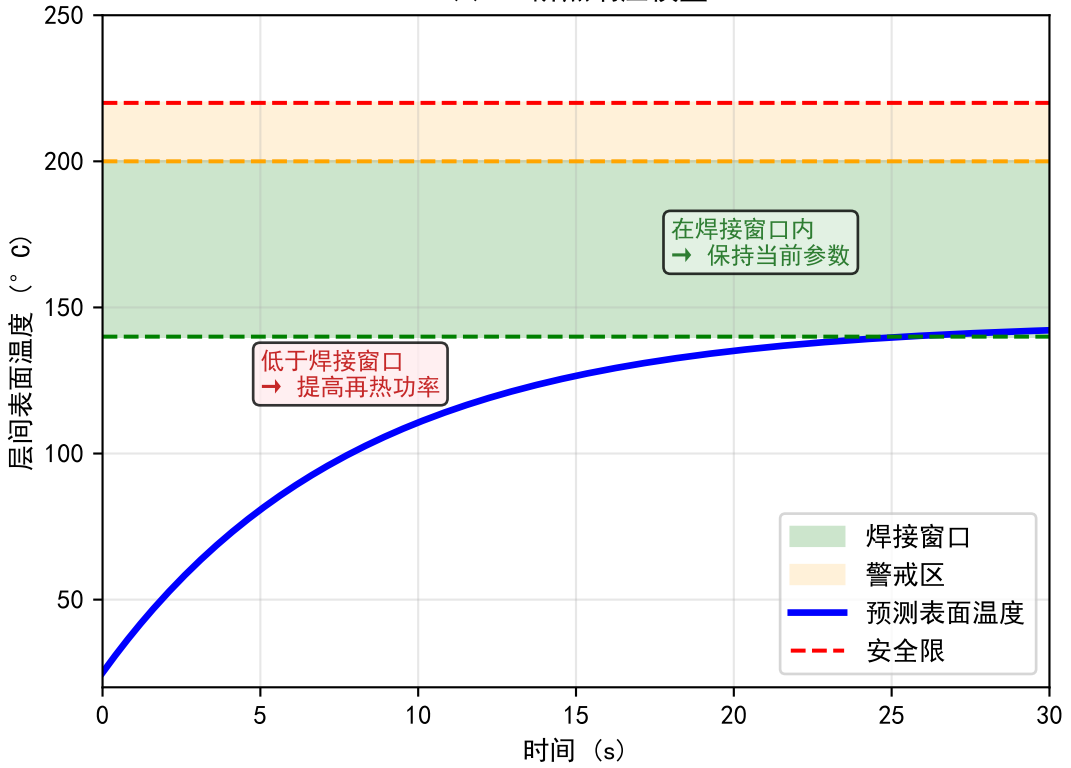
(b) 一阶热响应模型
