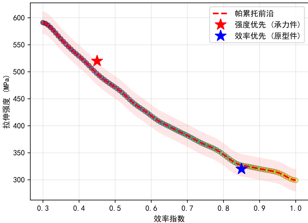
(c) 带优化偏好的帕累托前沿
