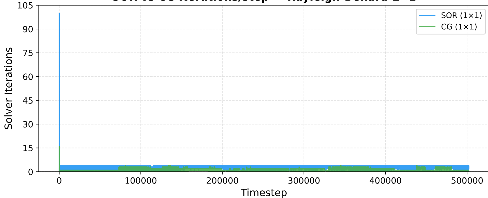
SOR vs CG iterations/step — Rayleigh-Bénard 1×1
