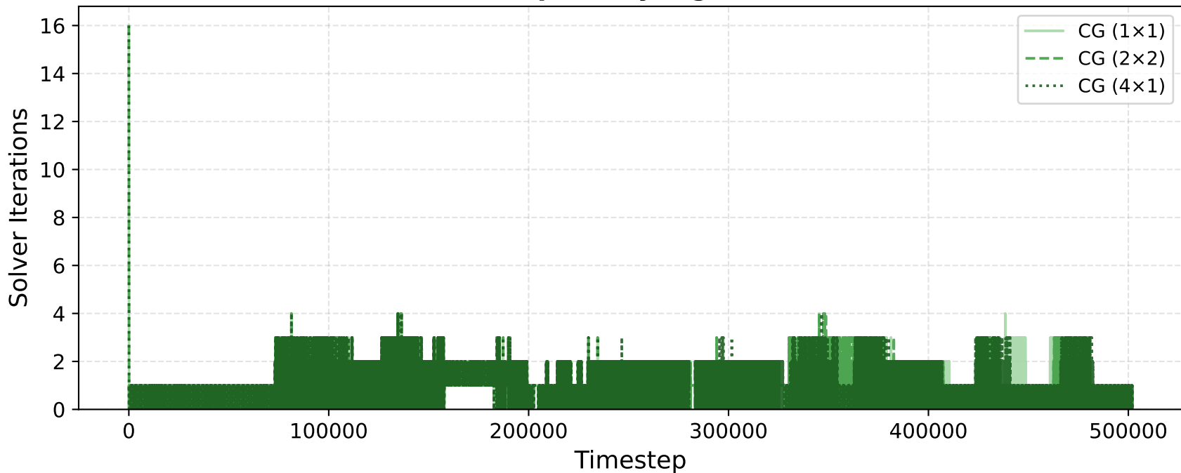
CG iterations/step — Rayleigh-Bénard (40×18)
