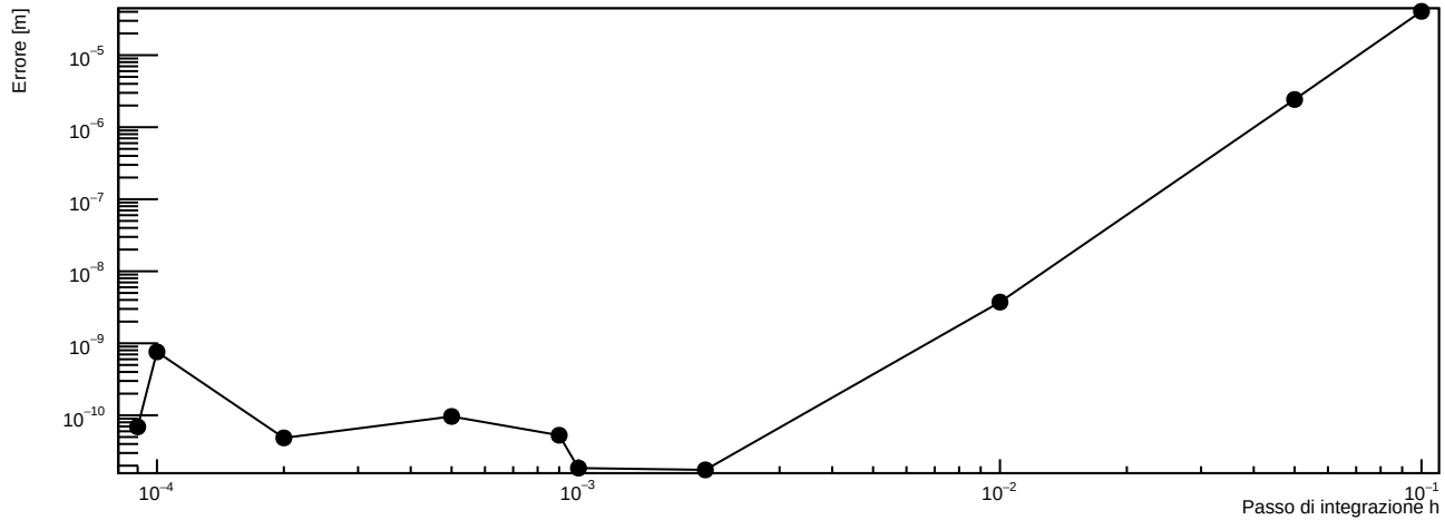
Errore con metodo di Runge-Kutta
