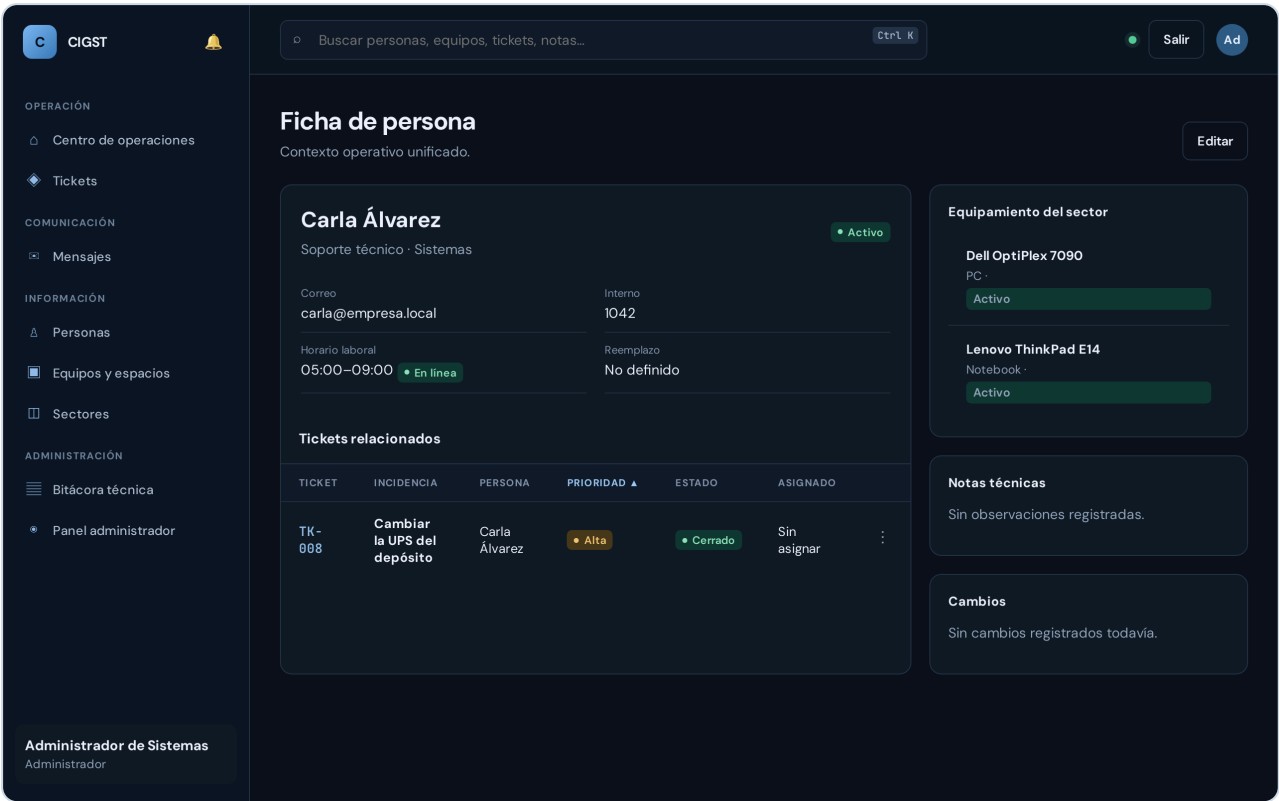
Ficha de persona, con su historial de Cambios a la derecha
