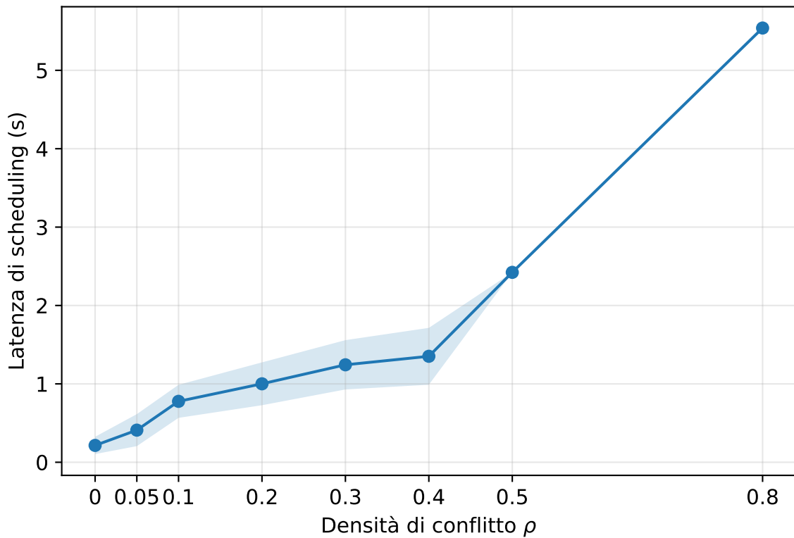
Latenza in funzione della densità di conflitto
