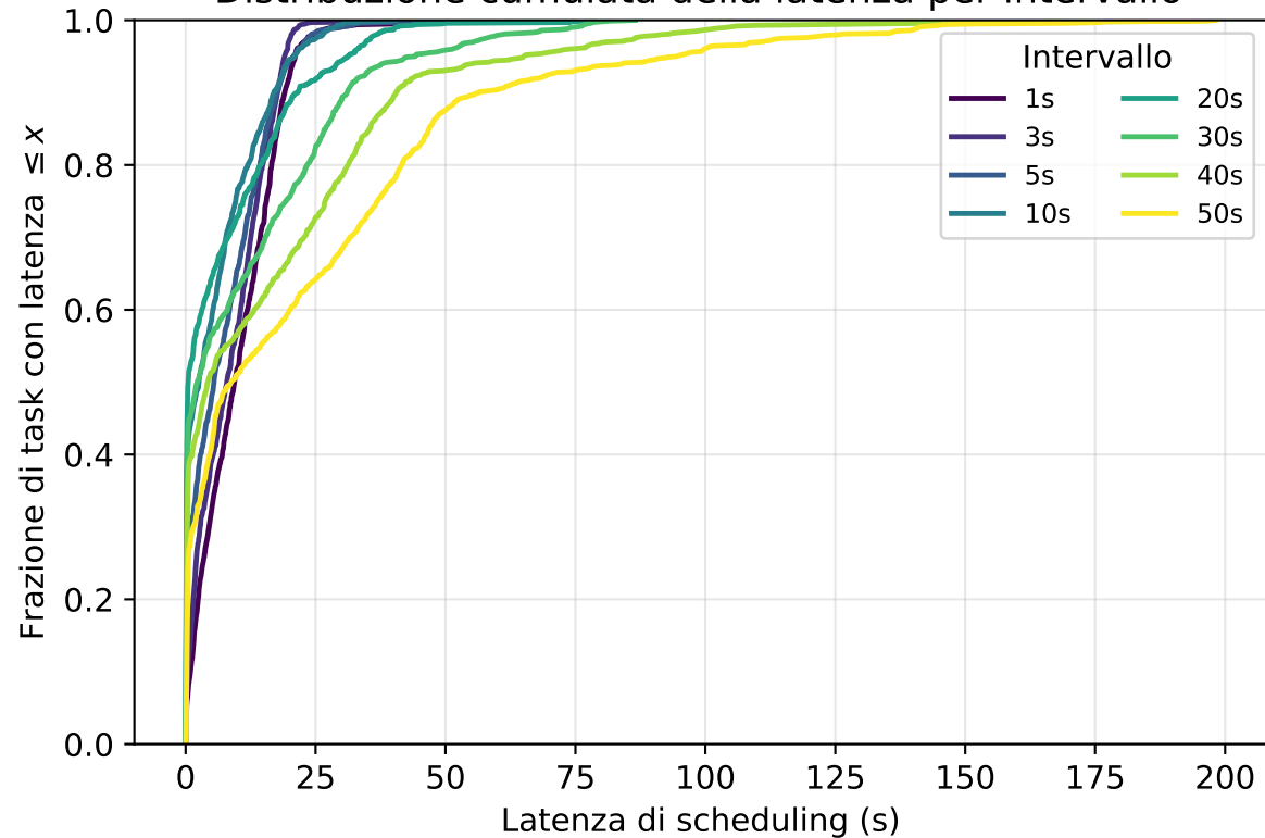
Distribuzione cumulata della latenza per intervallo
