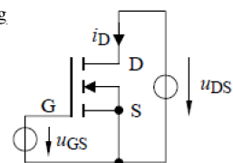
Messschaltung
