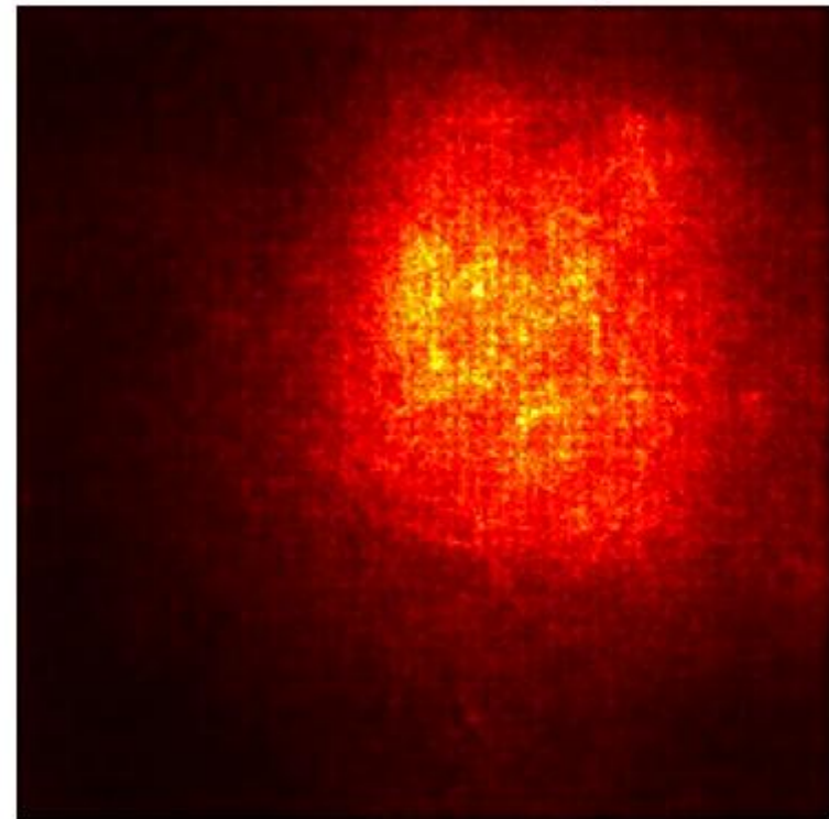
SmoothGrad Saliency
