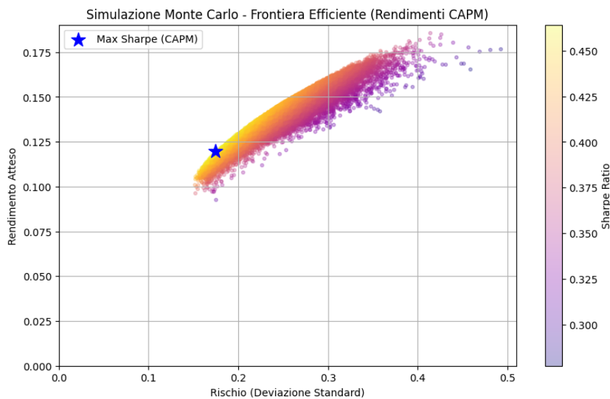
Figura 5.2: Simulazione Monte Carlo e Frontiera Efficiente (Rendimenti CAPM)
