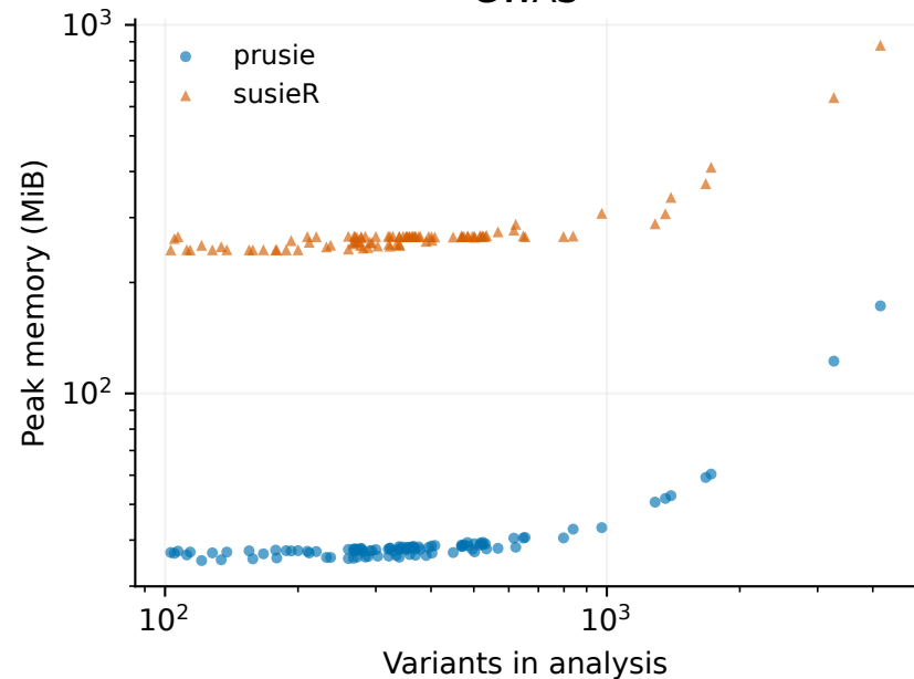
GWAS
