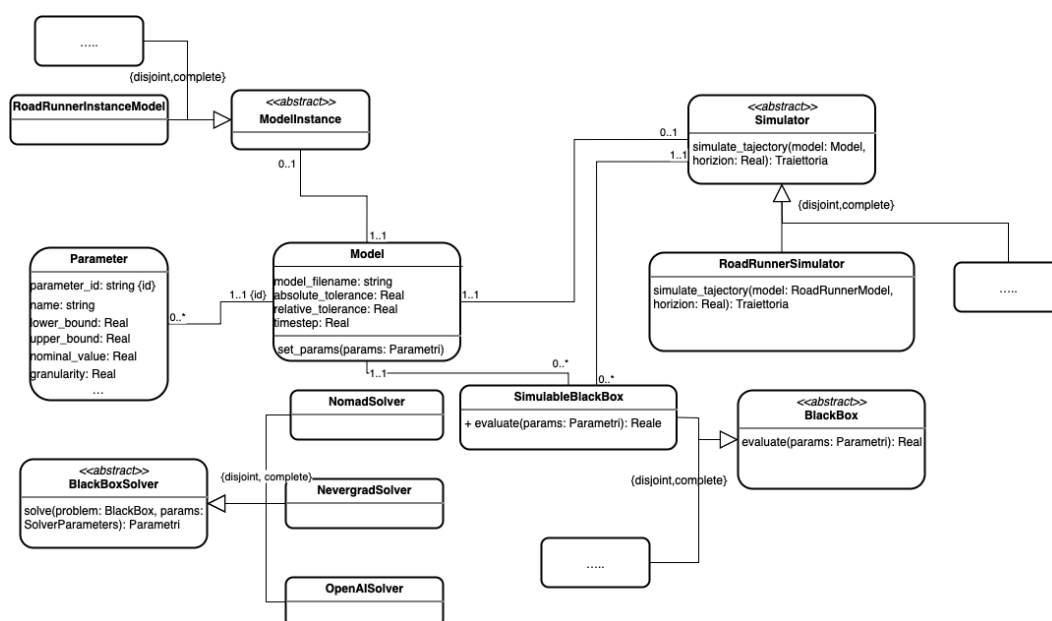
Figura 5.2 UML
