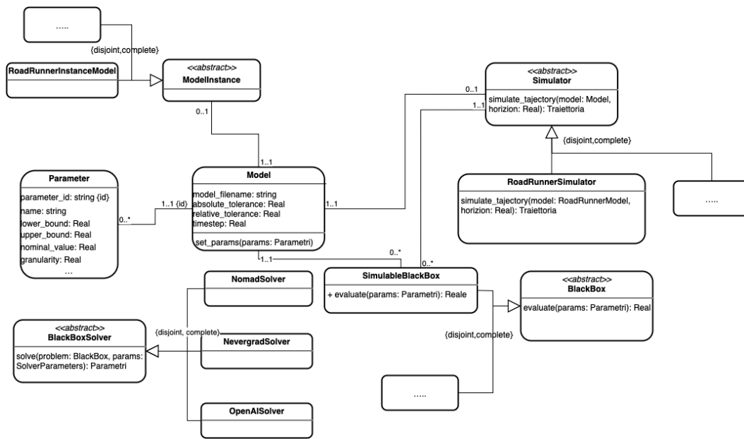
Figura 5.2 UML
