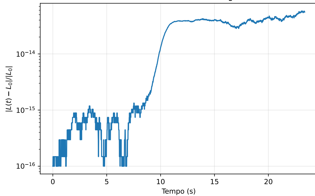
Erro relativo do momento angular
