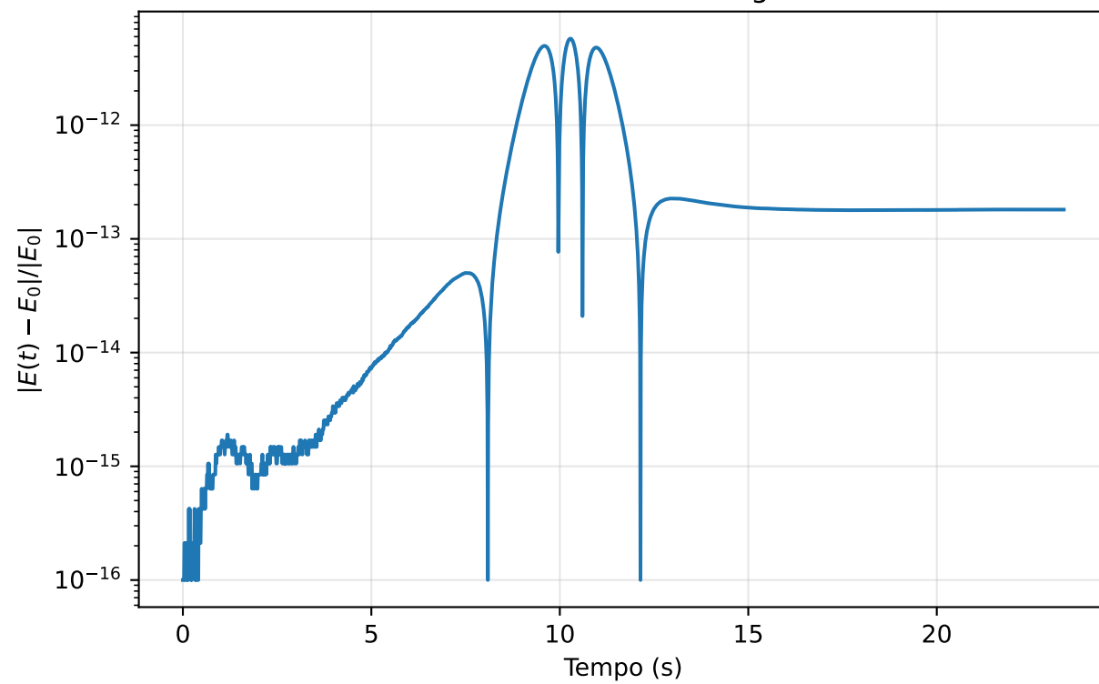
Erro relativo da energia
