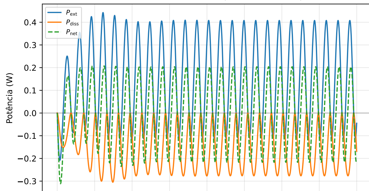
Potência — \omega = 1 rad/s (na ressonância)
