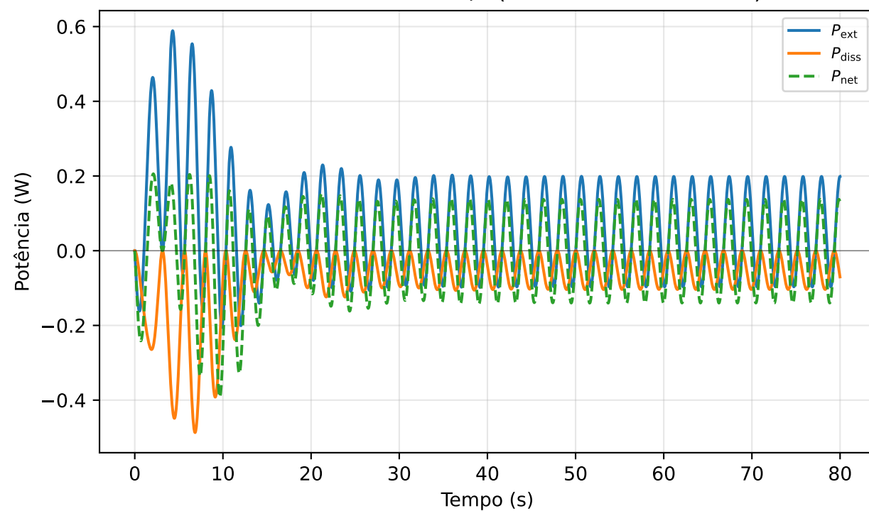
Potência — \omega = 1.5 rad/s (acima da ressonância)
