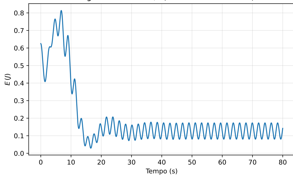
Energia — \omega = 1.5 rad/s (acima da ressonância)
