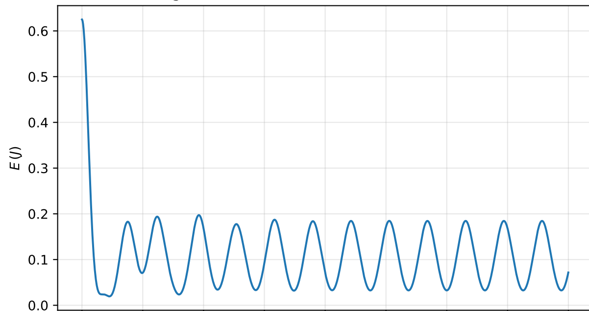
Energia — \omega = 0.5 rad/s (abaixo da ressonância)
