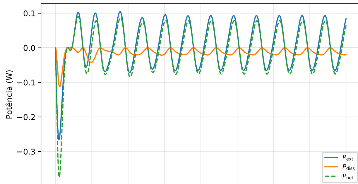
Potência — \omega = 0.5 rad/s (abaixo da ressonância)
