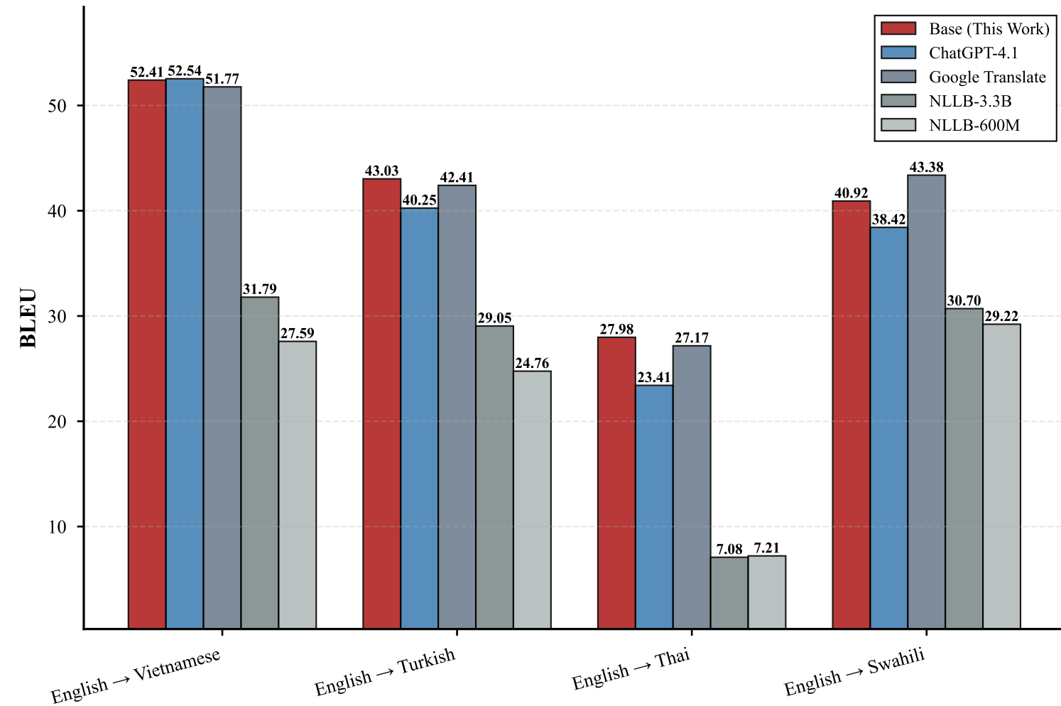
BLEU Score
