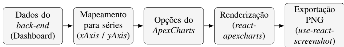
Figura 4.1 – Fluxo de geração de gráficos a partir dos dados de avaliação.
