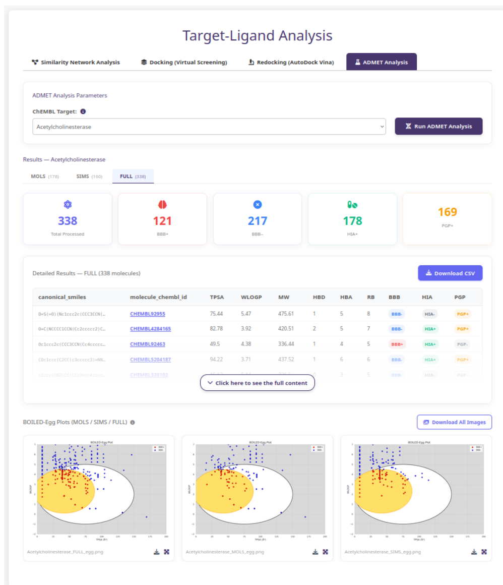
Figura 8: Tela da análise ADMET.
