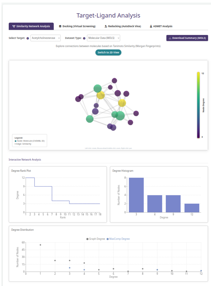
Figura 5: Tela da análise de redes de similaridade.
