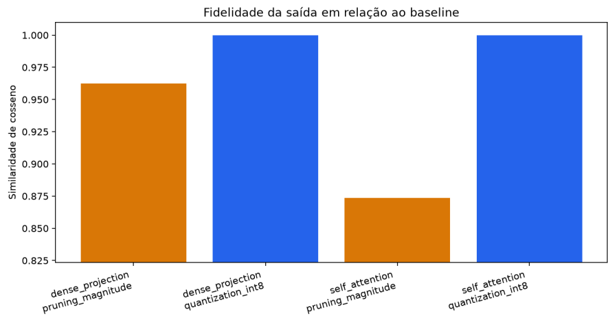
Figura 3.2: Qualidade numerica das saidas no diagnostico CPU v2.
