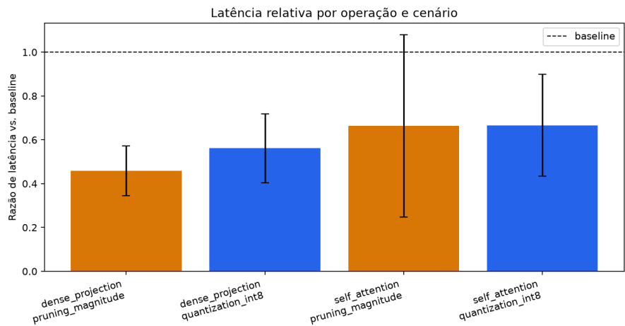
Figura 3.1: Diagnostico CPU v2. A figura valida a pipeline de analise, nao o desempenho do hardware alvo.
