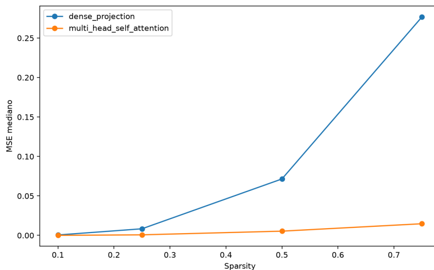
Figura 3.1: Degradação numerica por nível de sparsity na bateria sintetica v3.
