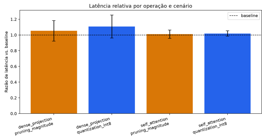
Figura 3.5: Latencia relativa do benchmark GPU v1, preservada como evidencia historica.
