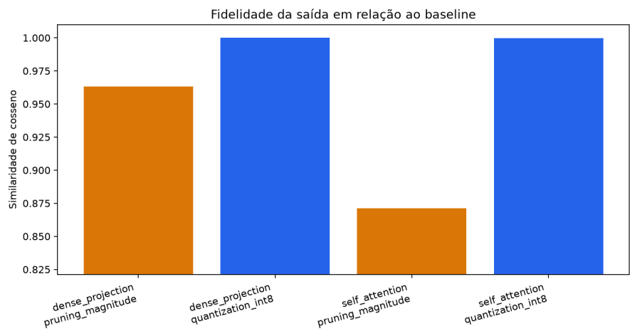
Figura 3.6: Fidelidade numerica do benchmark GPU v1.
