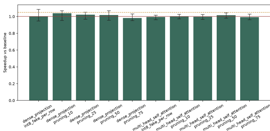
Figura 3.2: Speedup mediano e intervalos bootstrap de 95%; nenhum candidato satisfaz o criterio de ganho fisico.
