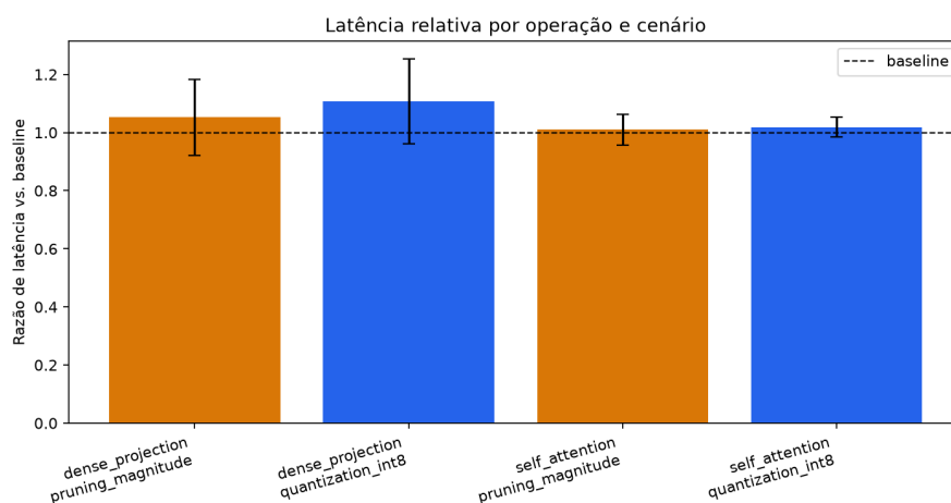
Figura 3.3: Latencia relativa do benchmark GPU v1, preservada como evidencia historica.
