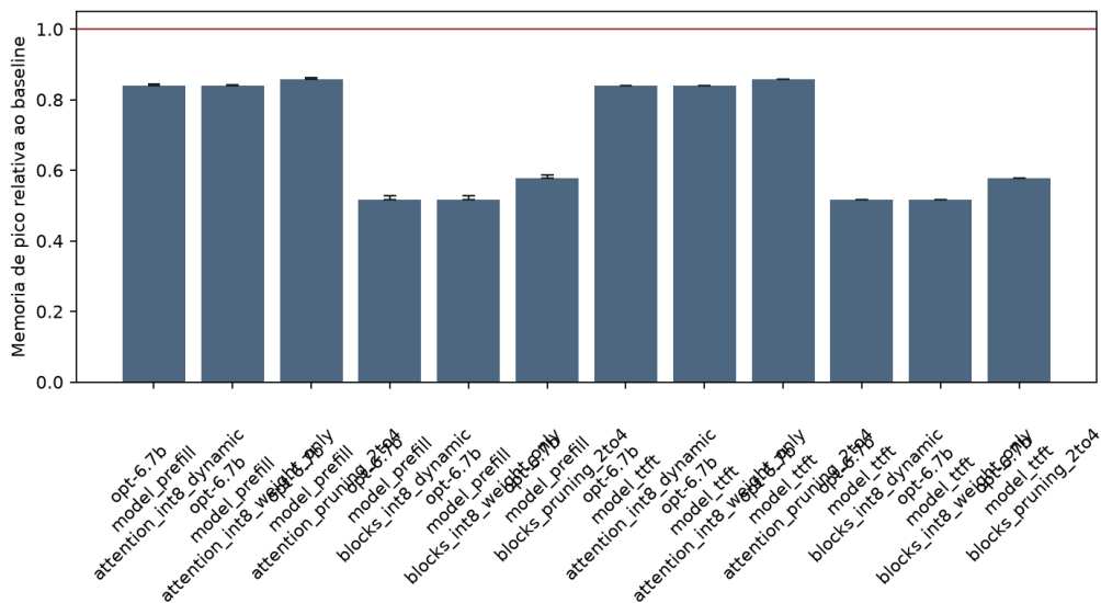
Figura 3.10: Memoria de pico relativa na extensao OPT-6.7B.
