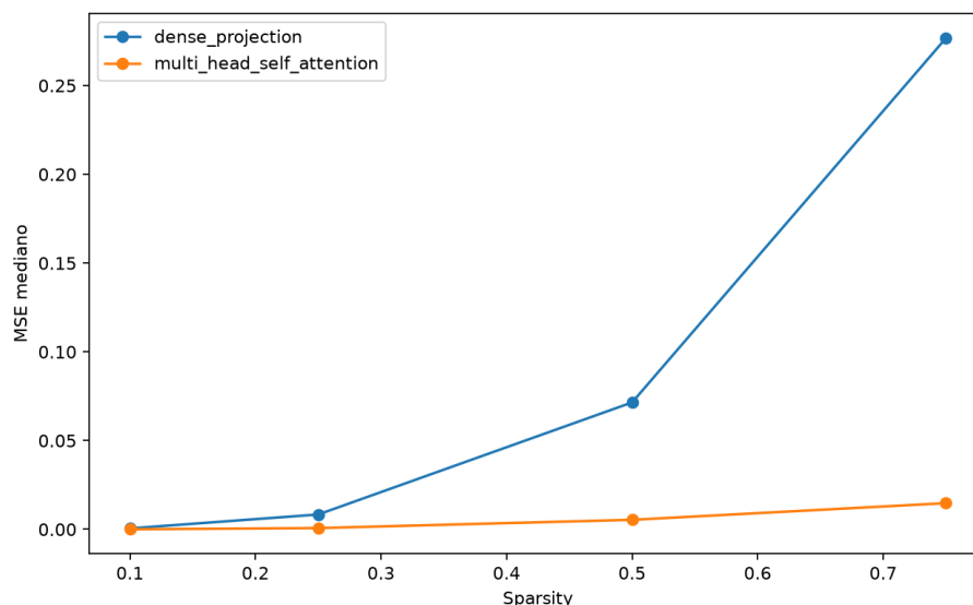
Figura 3.1: Degradação numérica por nível de sparsity na bateria sintética v3.
