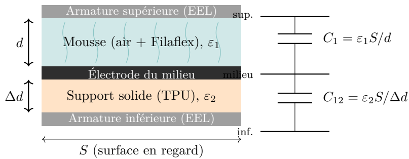
Figure 5. Second capteur à électrodes superposées (schéma) : la cellule inférieure C_2 , mesurée entre l'armature supérieure et l'armature inférieure, correspond à la mise en série de la mousse ( C_1 ) et du support solide ( C_{12} ), soit 1/C_2 = 1/C_1 + 1/C_{12} .
