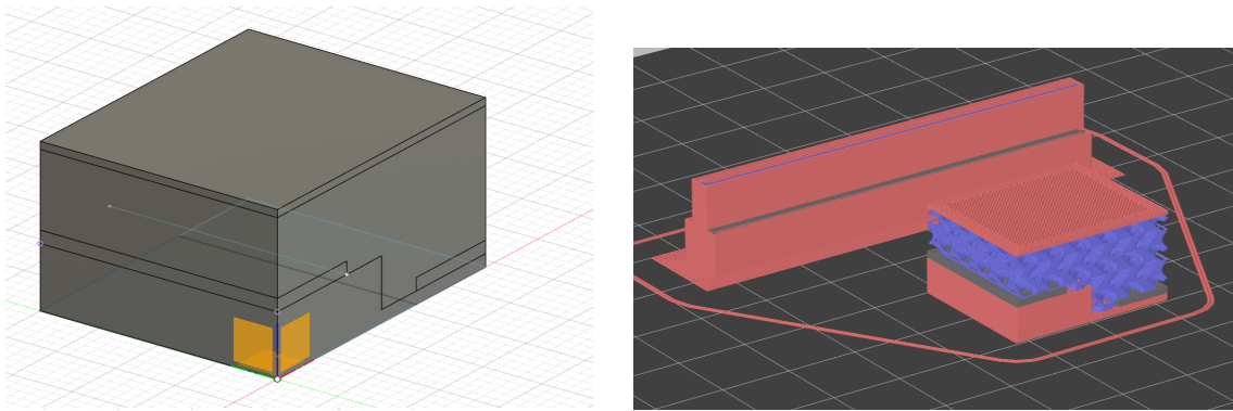
Figure 3. Différentes étapes de la pièce : perspective cavalière en CAO (gauche) ; vue dans le slicer après découpage (droite). La pièce allongée visible à côté du capteur est la tour de nettoyage, utilisée pour purger les résidus de filament lors des changements de matériau.
