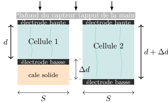
Figure 2. Premier prototype (V1) : deux cellules côte à côte, partageant le même diélectrique en mousse ( \varepsilon ) et la même surface S .
