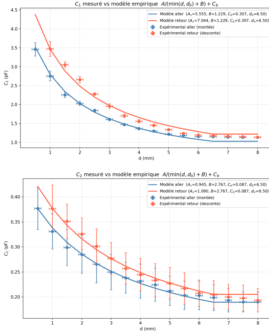
Figure 11. C_1 et C_2 en fonction de d . Avec le fit, on pose \min(d, d_0) car la compression ne démarre pas à 8 mais au moment où la mousse s'écrase, c'est-à-dire d = 6,5 .
