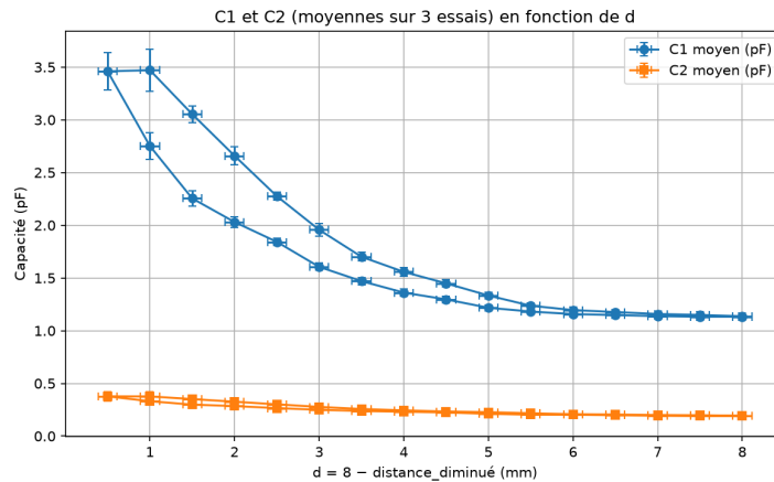
Figure 10. Mise en évidence du phénomène d’hystérésis : pour un même écartement, la capacité diffère selon que la mousse est en cours de compression ou de relâchement. Ici, l’échelle de valeurs est cohérente car, grâce au second membre de l’égalité, 1/C_2 > 1/C_1 . C_1 et C_2 moyens correspondent aux valeurs moyennes pour 3 mesures en fonction de d .
