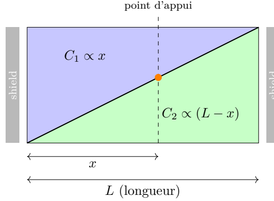
Figure 13. Capteur de position à deux triangles capacitifs complémentaires, avec blindage latéral. La surface de C_1 croît avec x , celle de C_2 décroît.
