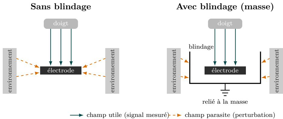
Figure 7. Blindage relié à la masse (type Faraday). Sans blindage (gauche) Avec blindage (droite)
