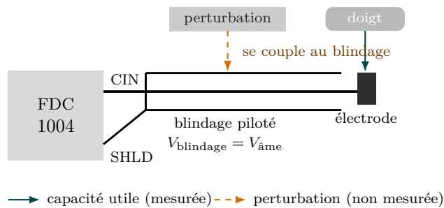
Figure 8. Blindage actif piloté (sorties SHLD de la FDC 1004).
