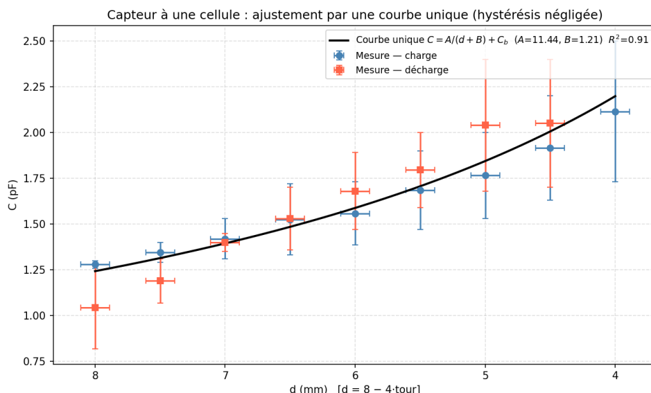
Figure 12. Capteur à une cellule unique : capacité mesurée (deux essais moyennés, branches de charge et de décharge) en fonction de d = 8 - 4 \text{ tour} , ajustée par une unique courbe C = A/(d + B) + C_b . Les barres d'erreur, très larges, traduisent le caractère improvisé du montage ; les points de charge et de décharge se confondent en leur sein.
