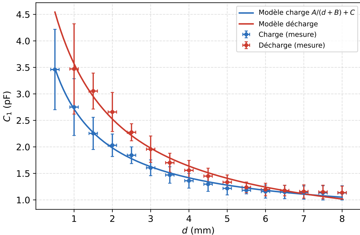
C_1 : ajustement empirique A/(d + B) + C par branche
