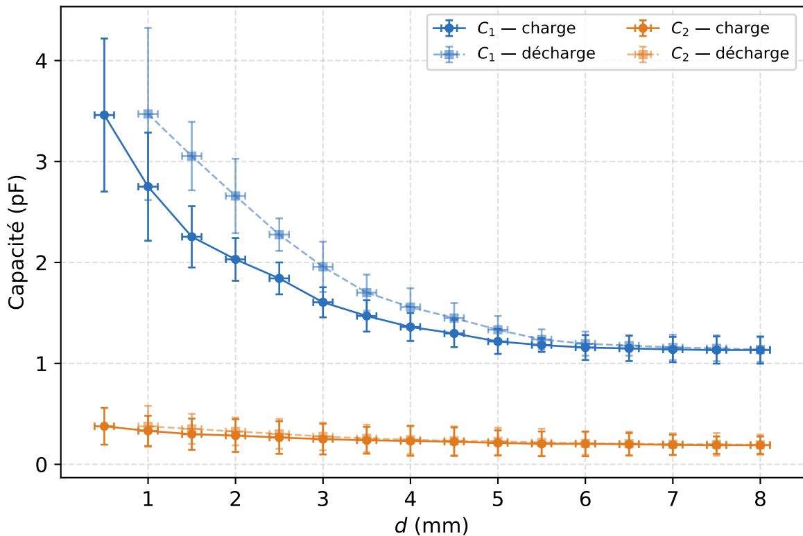
Capacités mesurées en fonction de l'écartement (barres : U_{95} )
