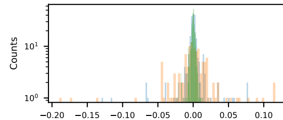
fDcaXY2
