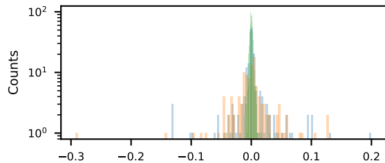
fDcaXY1
