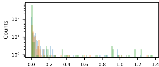
fDCAxyzTrk0KF
