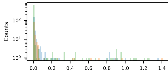
fPairDCAxyz
