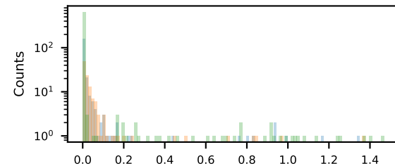
fDCAxyzTrk1KF
