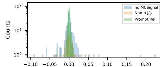
fPairDCAxy
