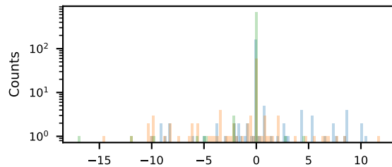
fDcaZ1
