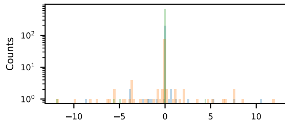
fDcaZ2
