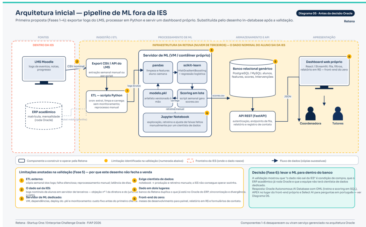
Figura 10 — Arquitetura inicial (Fases 1-5): ETL externo, servidor de ML e dashboard fora do banco da IES
