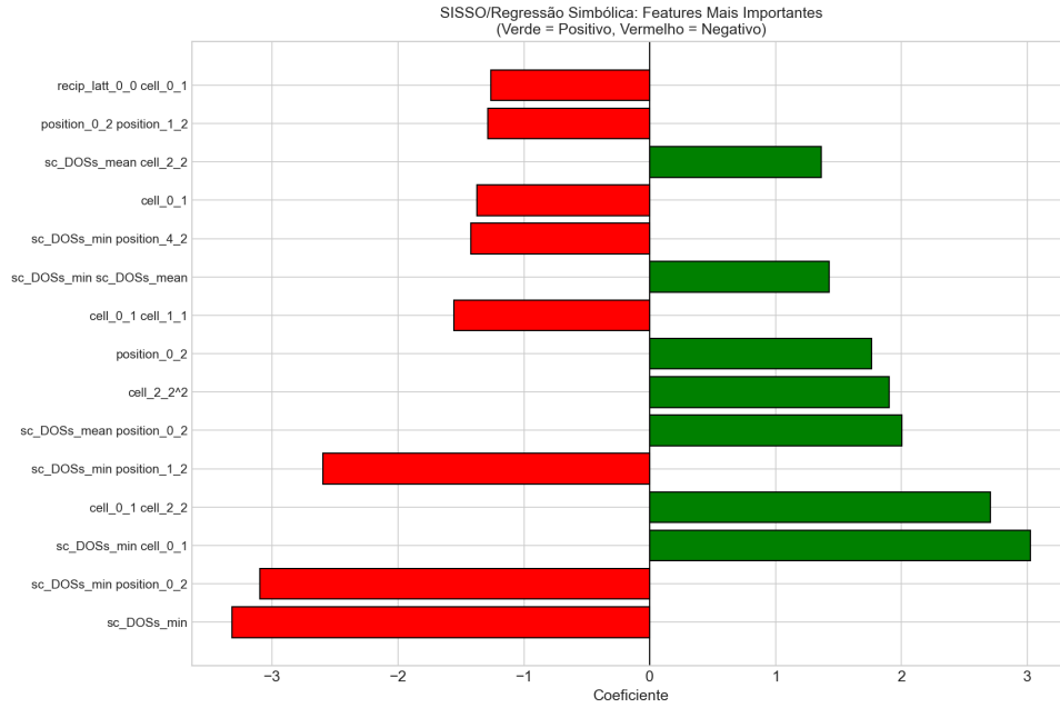
Figura 5.15: Coeficientes da equação descoberta pelo SISSO. A dominância de termos envolvendo a densidade de estados ( sc\_DOSs\_min ) é evidente.
